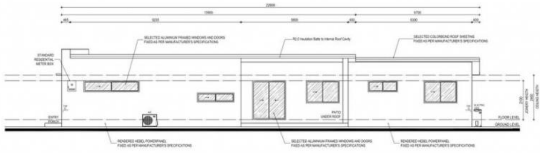
ELEVATION 2 1:100
