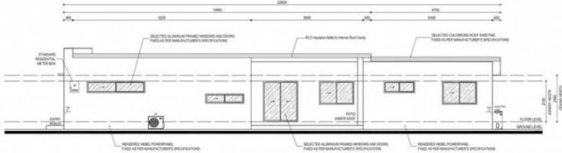
ELEVATION 2 1:100
